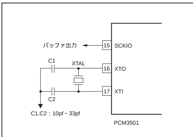
図3. クリスタル発振接続例
