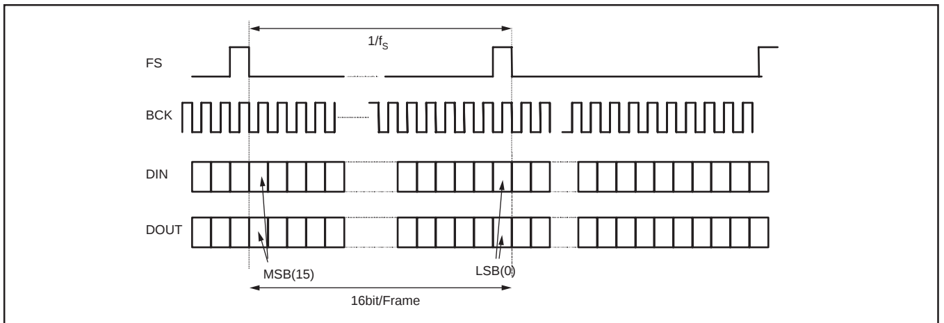
図10. シリアル・インターフェース・フォーマット
