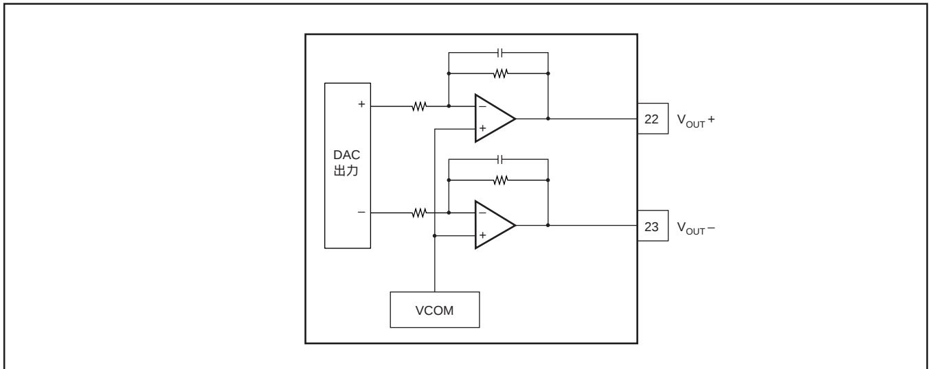
図2. PCM3501 DAC出力部等価回路
