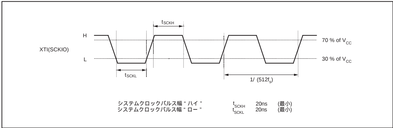
図5. 外部システムクロック入力タイミング規定
