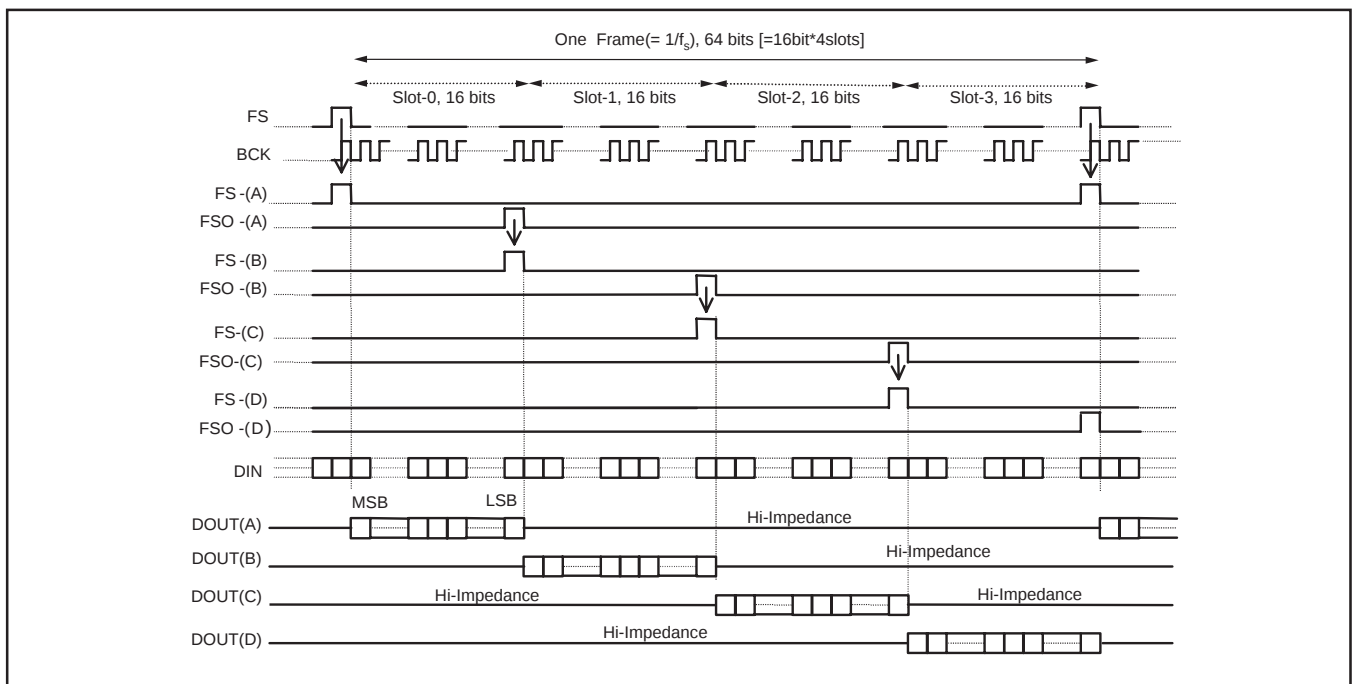
図14. タイムスロット動作タイミング
