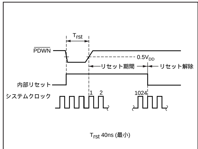
図7. パワーダウンおよび外部リセット・タイミング
