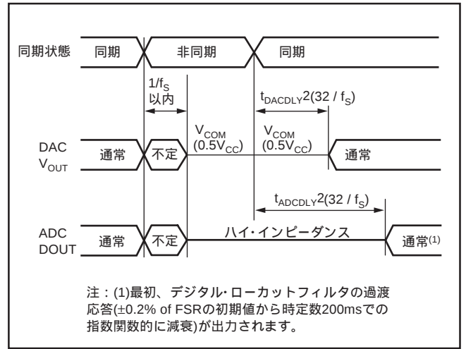
図9. 同期/非同期時のADC/DAC出力
