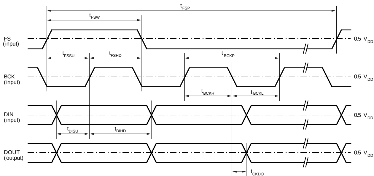
図11. シリアル・インターフェース・タイミング規定(マスター・モード)
