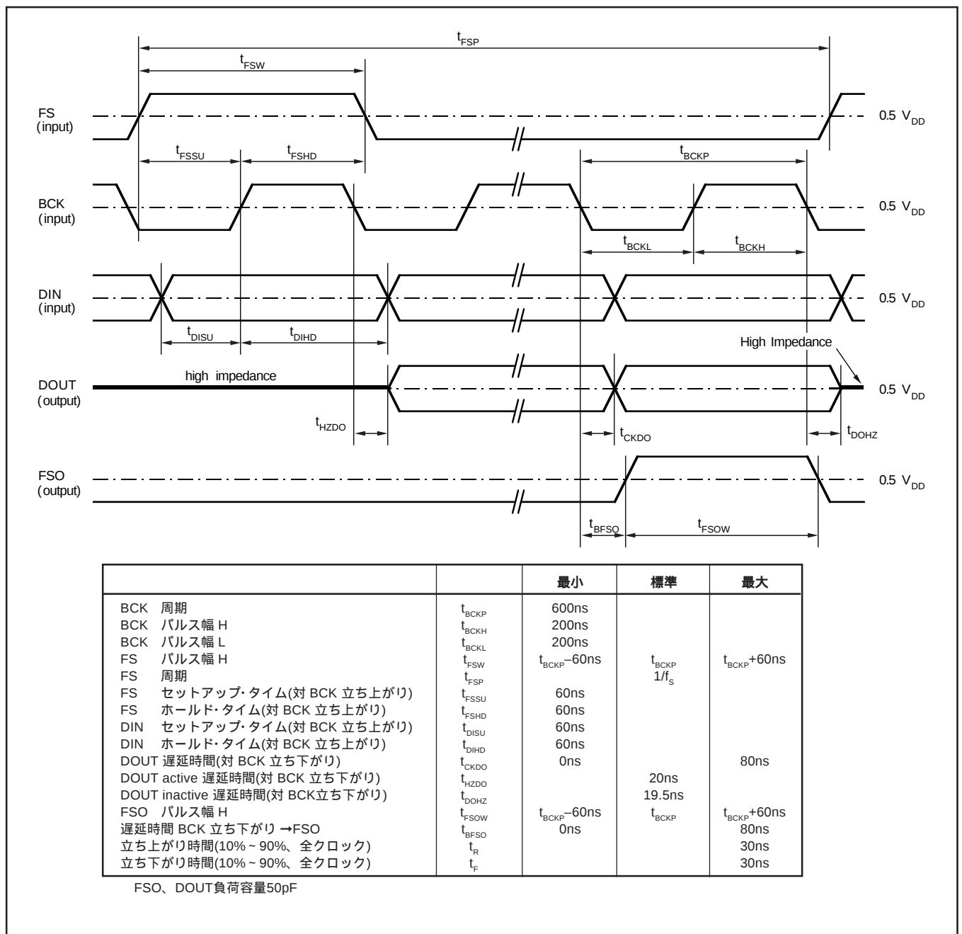
図16. タイムスロット動作タイミング規定(スレープ・モード)
