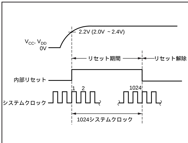
図6. パワーオン・リセット・タイミング
