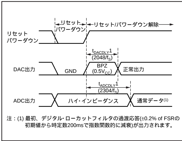
図8. リセット・パワーダウでのADC/DAC出力
