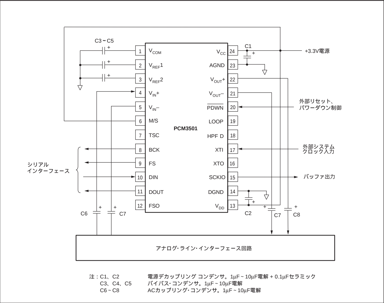
図16. PCM3501基本接続図
