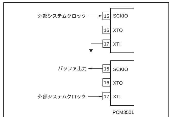
図4. 外部システムクロック入力接続例
