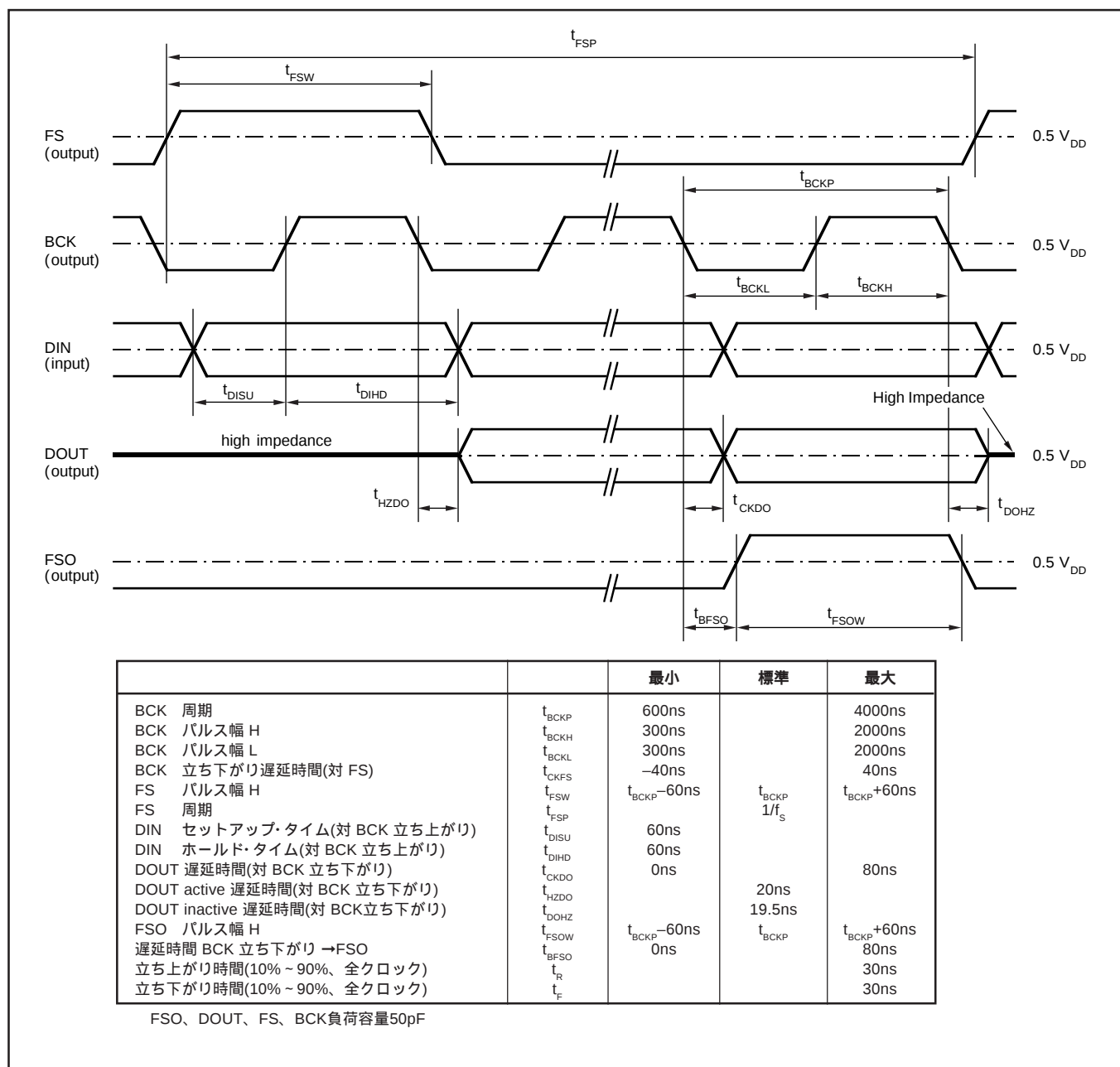
図15. タイムスロット動作タイミング規定(マスター・モード)
