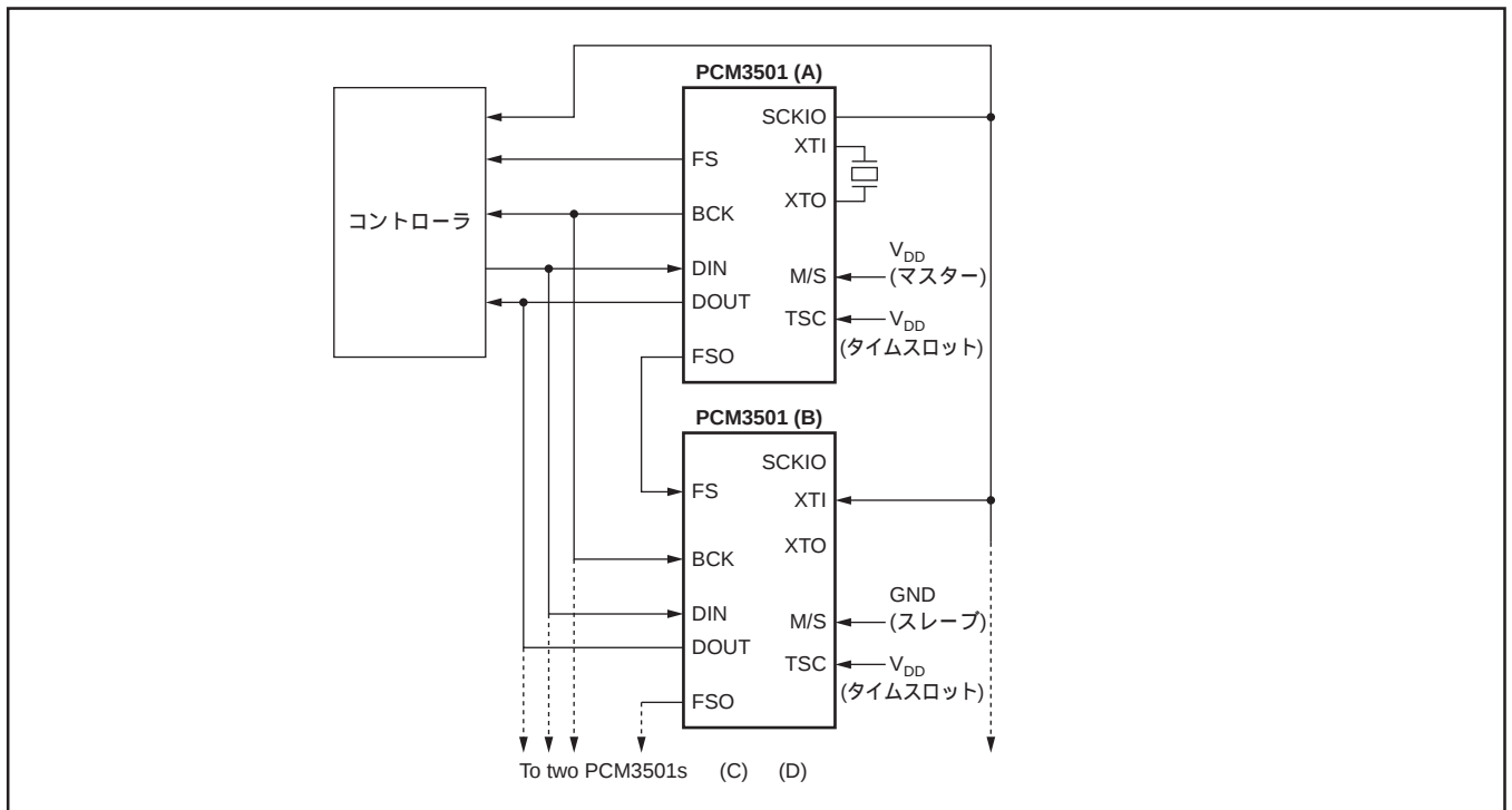
図13. タイムスロット動作接続例
