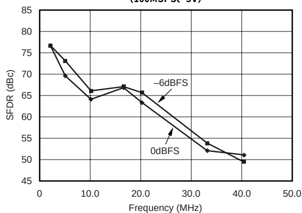
スプリアスフリー・ダイナミック・レンジ対 f_{\text{OUT}} (100MSPS、3V)
