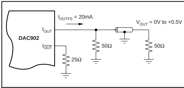
図6. 二重終端した50Ωケーブルの直接ドライブ
