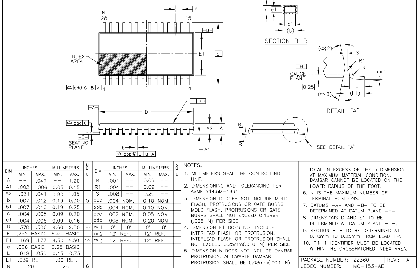
パッケージ番号360-28ピンTSOP
