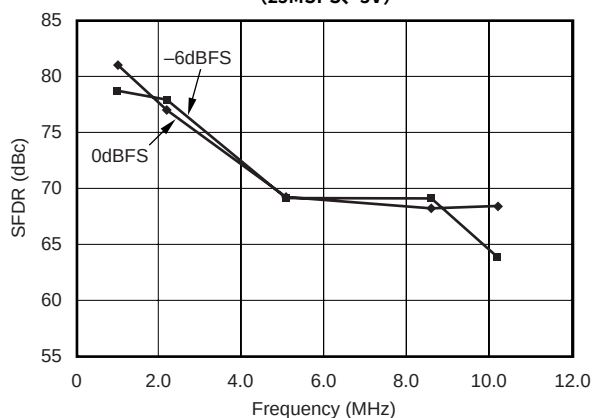
スプリアスフリー・ダイナミック・レンジ対 f_{\text{OUT}} (25MSPS、3V)
