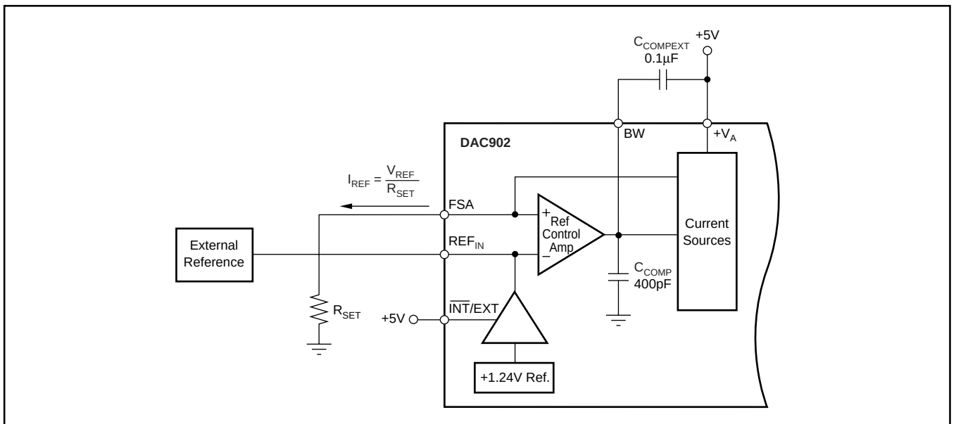
図8. 外部リファレンスの構成
