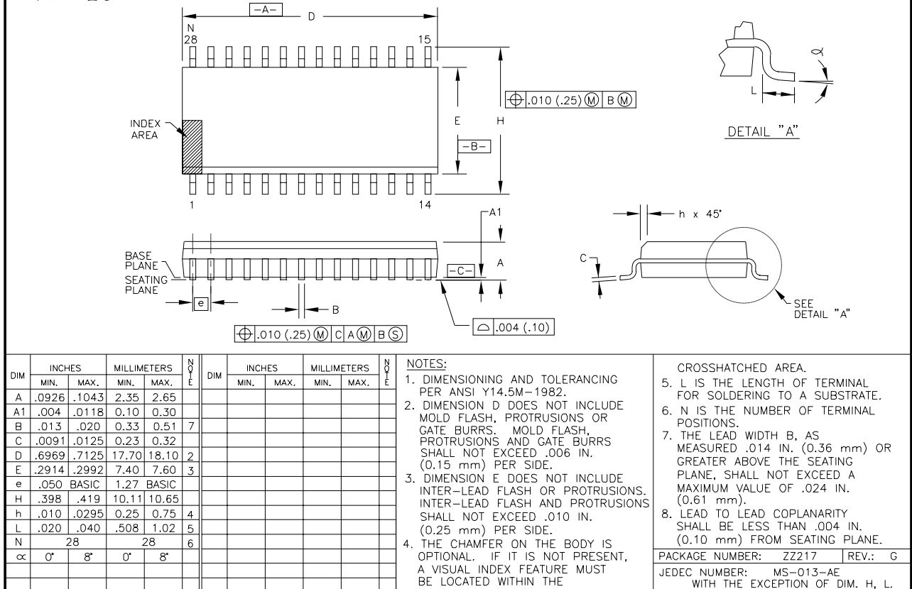
パッケージ番号217-28ピンSOP
