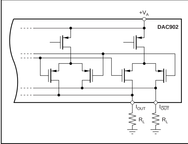
図2. 等価アナログ出力
