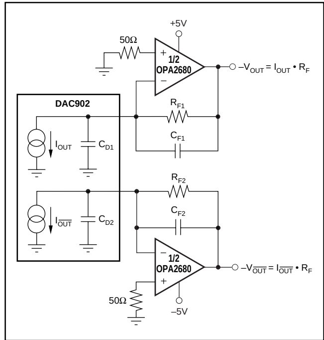
図5. デュアル・タイプの電圧帰還アンプOPA2680で構成した差動トランスインピーダンス・アンプ
