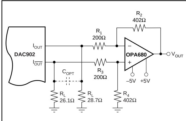
図4. 差動アンプによる差動からシングルエンドへの変換とAC結合
