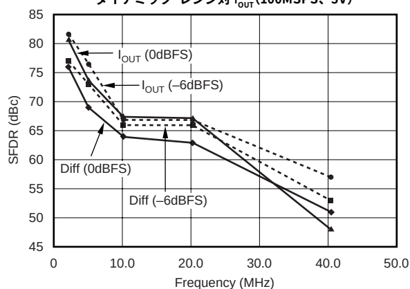
差動対シングルエンドスプリアスフリー・ ダイナミック・レンジ対 f_{\text{OUT}} (100MSPS、3V)
