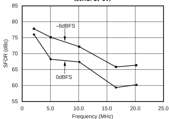
スプリアスフリー・ダイナミック・レンジ対 f_{\text{OUT}} (50MSPS、3V)
