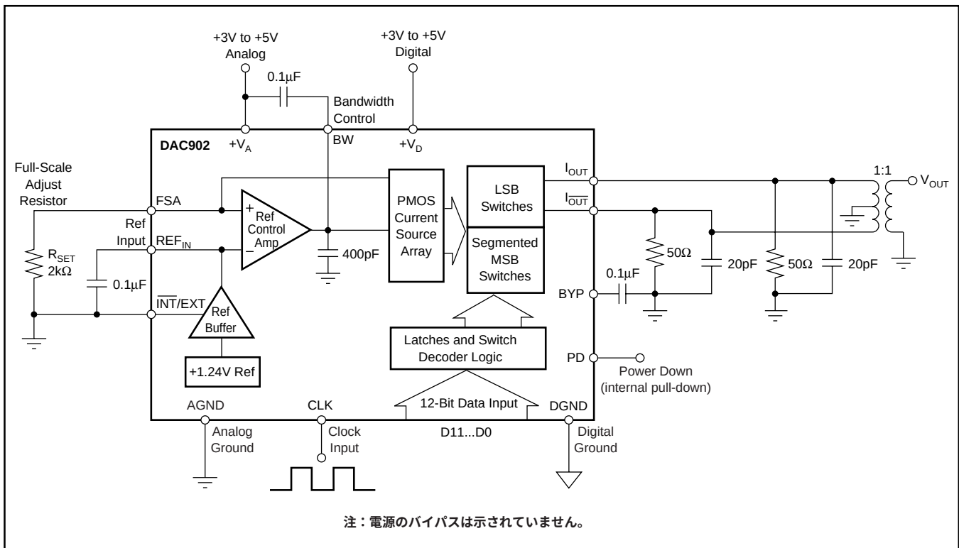
図1. DAC902の機能ブロック図
