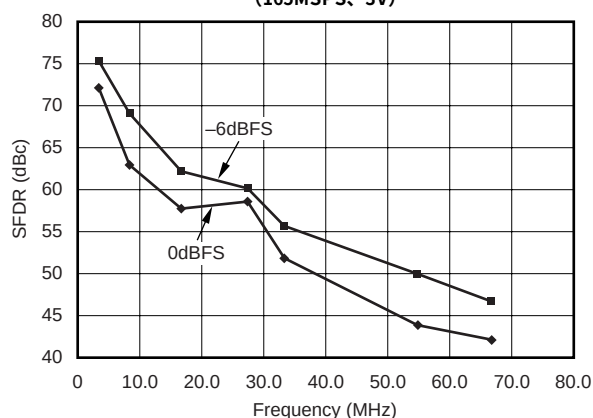
スプリアスフリー・ダイナミック・レンジ対 f_{\text{OUT}} (165MSPS、3V)
