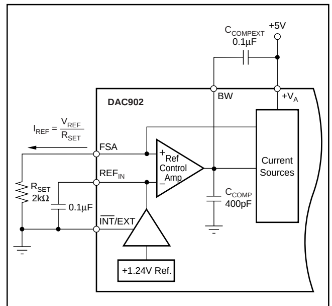
図7. 内部リファレンス構成
