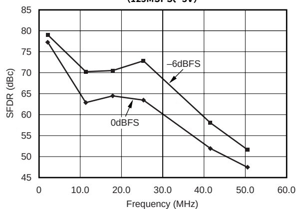
スプリアスフリー・ダイナミック・レンジ対 f_{\text{OUT}} (125MSPS、3V)
