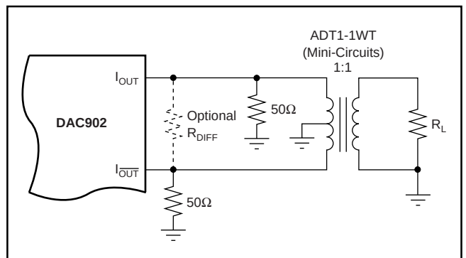
図3. RFトランスを使用した差動出力構成
