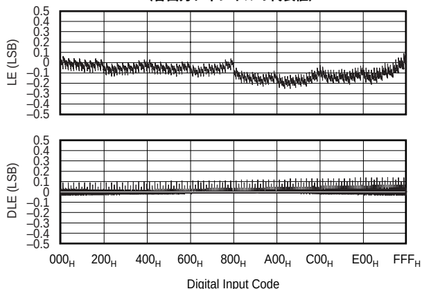
直線性誤差および微分直線性誤差対コード 1チャンネル：-40°C (各出力チャンネルの代表値)
