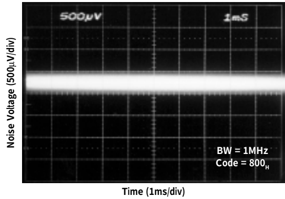
広帯域雑音
