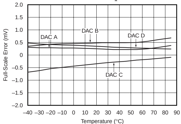
フルスケール誤差対温度 (コードFFF H )
