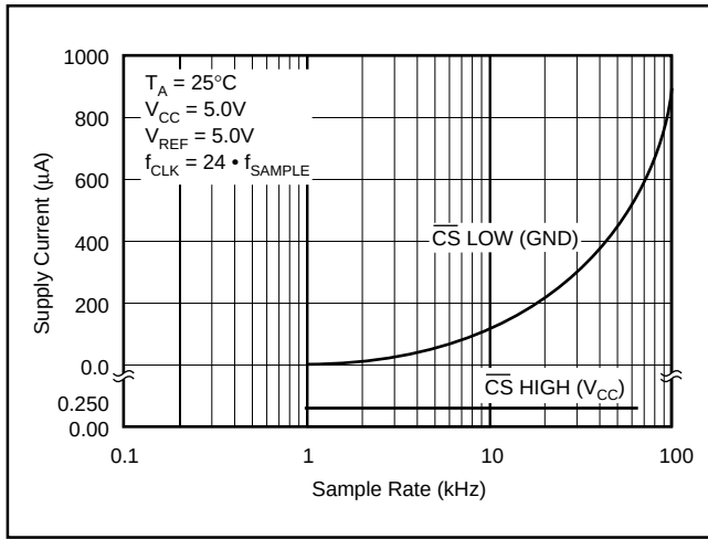
図7. \overline{CS} が「ハイ」のときのシャットダウン電流はクロックに関係なく通常は50nAであり、 \overline{CS} が「ロー」のときのシャットダウン電流はサンプリング・レートによって変化する
