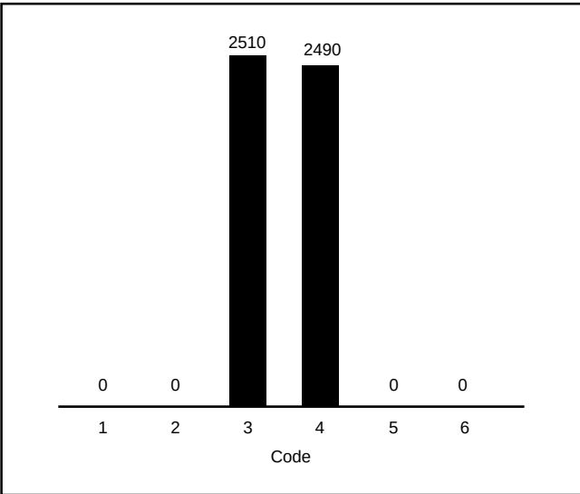
図1. DC入力の変換5,000回のヒストグラム(コード・トランジション)
