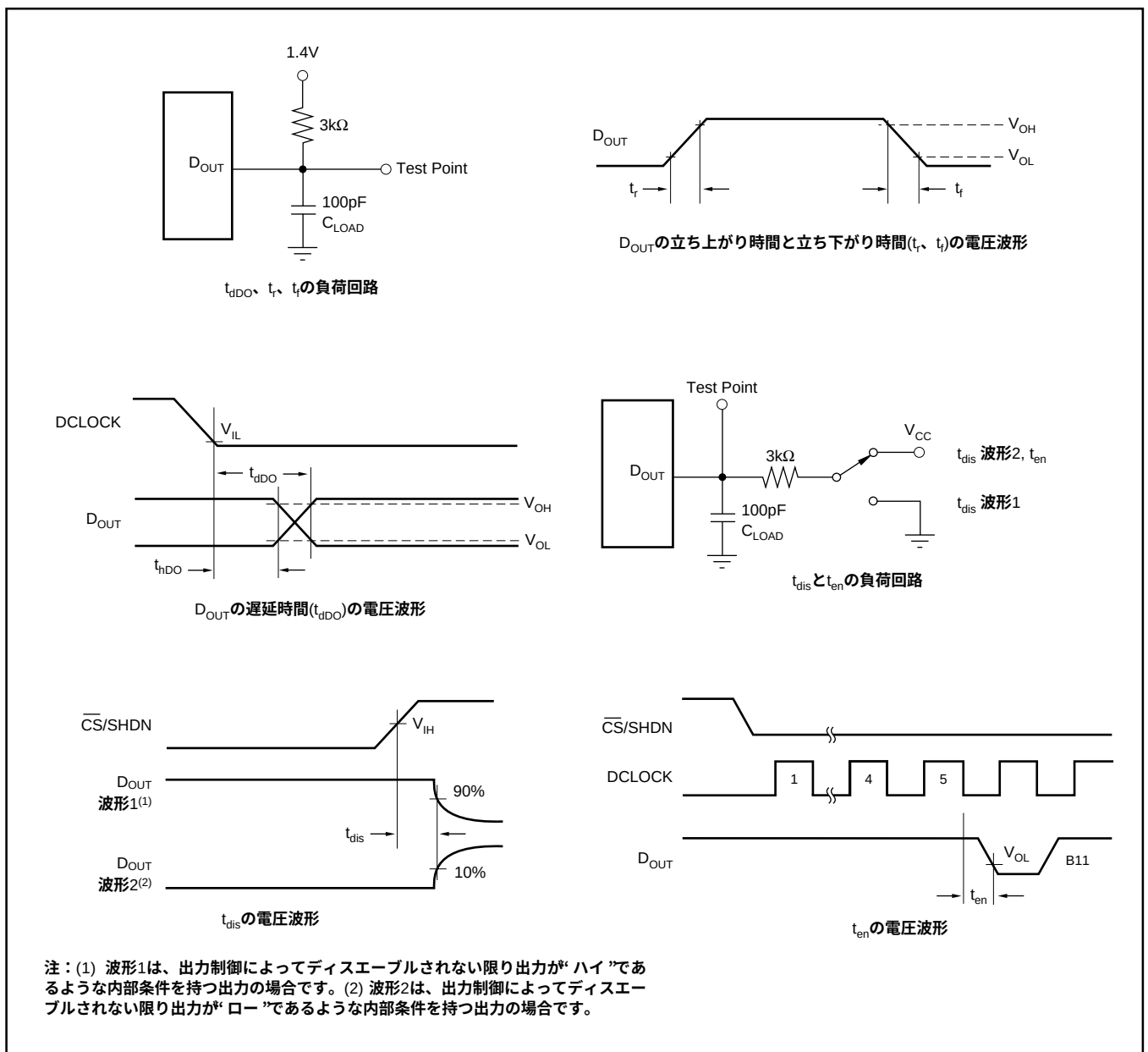
図4. 表 I のパラメータに関するタイミング図とテスト回路
