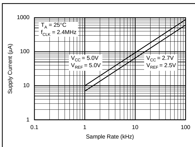
図5. f_{CLK} を可能な限り最大のレートに維持することにより、電源電流はサンプリング・レートに対してリニアに減少する
