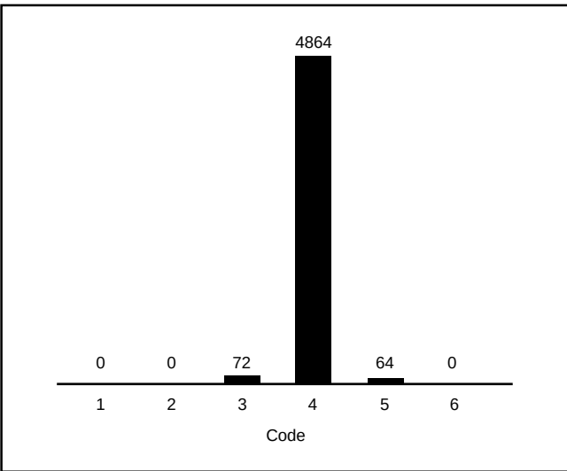
図2. DC入力の変換5,000回のヒストグラム(コード・センター)
