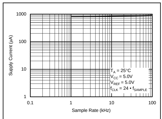
図6. f_{CLK} をスケーリングすると、電源電流はサンプリング・レートに対してわずかにしか減少しない
