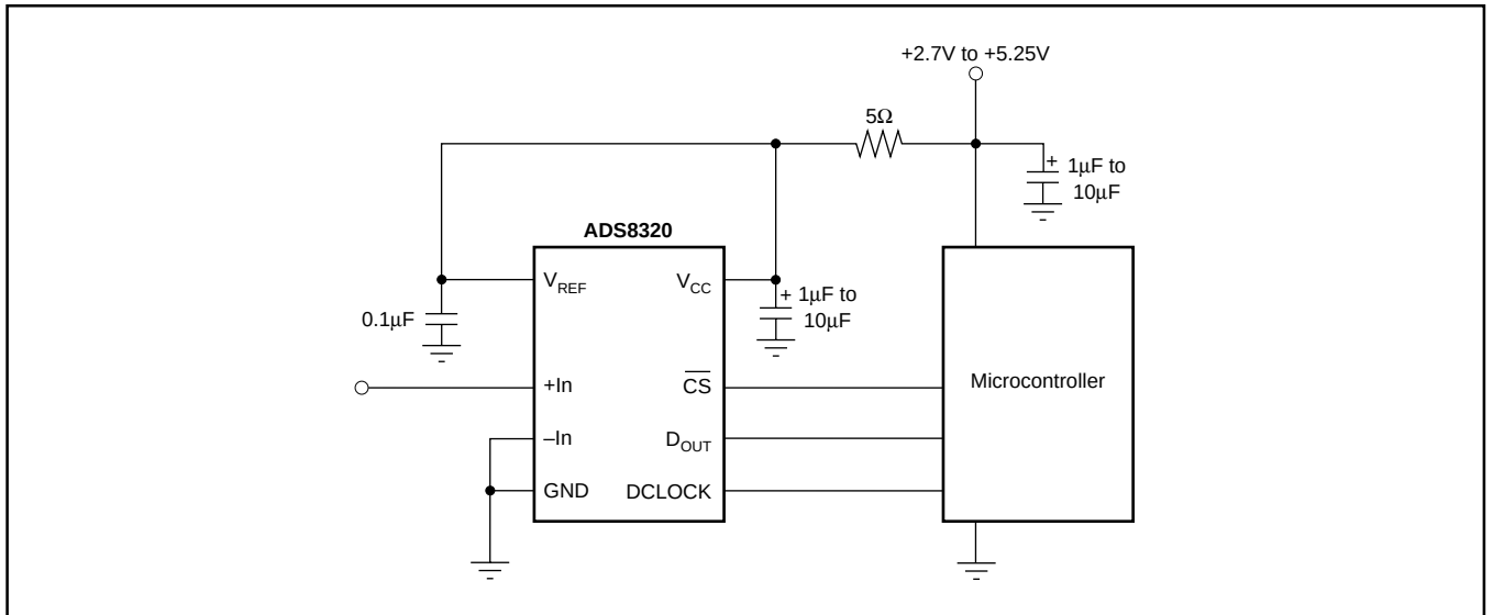
図8. 基本的なデータ・アキュイジション・システム
