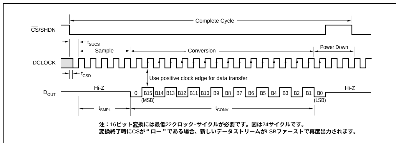
図3. ADS8320の基本タイミング図
